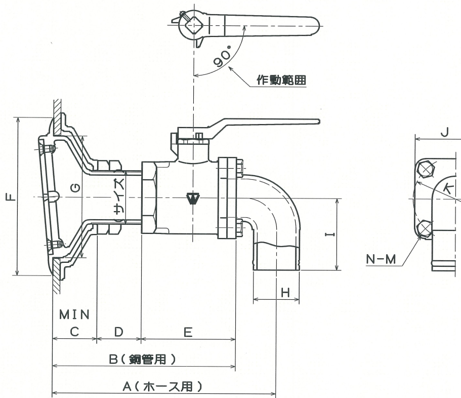
TA型 高速吸水式キングストン
